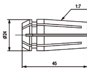
Collets Taper 1 : 7
